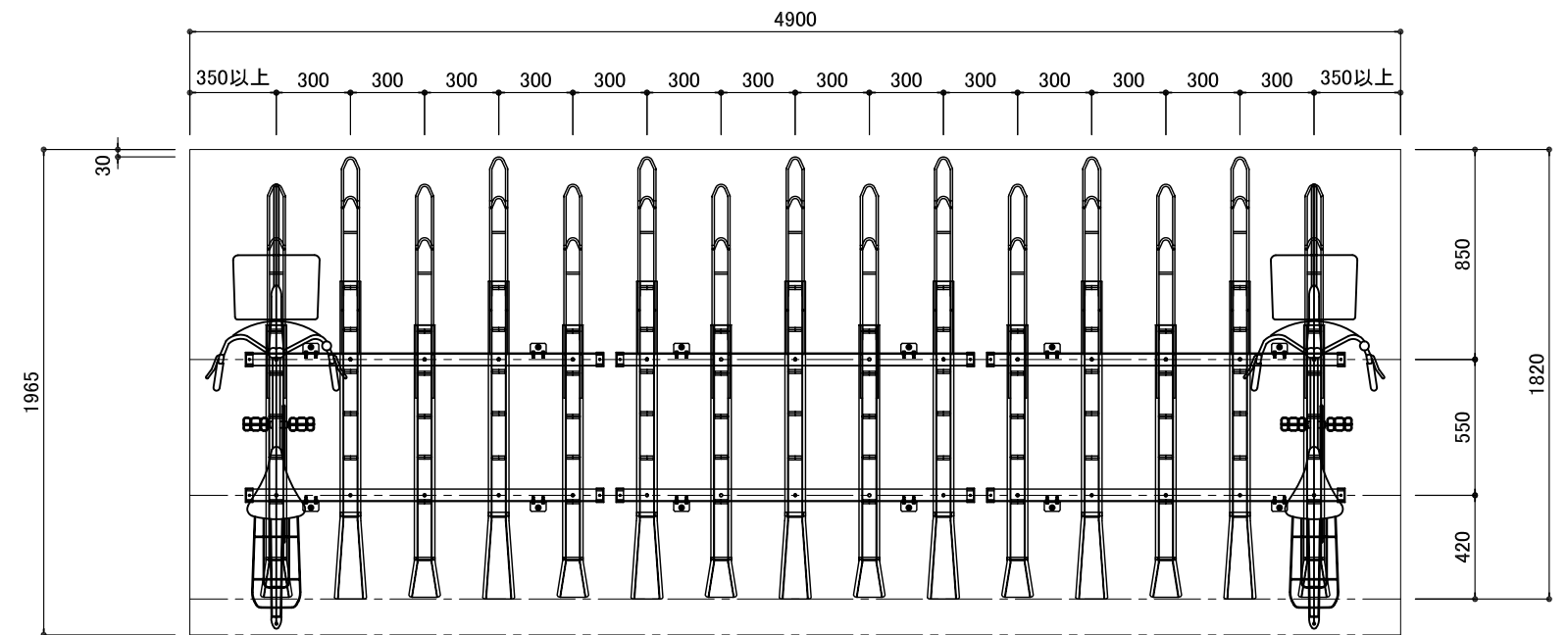
平面図 S=1/30
