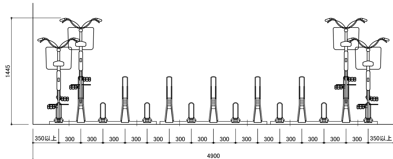
立面図 S=1/30
