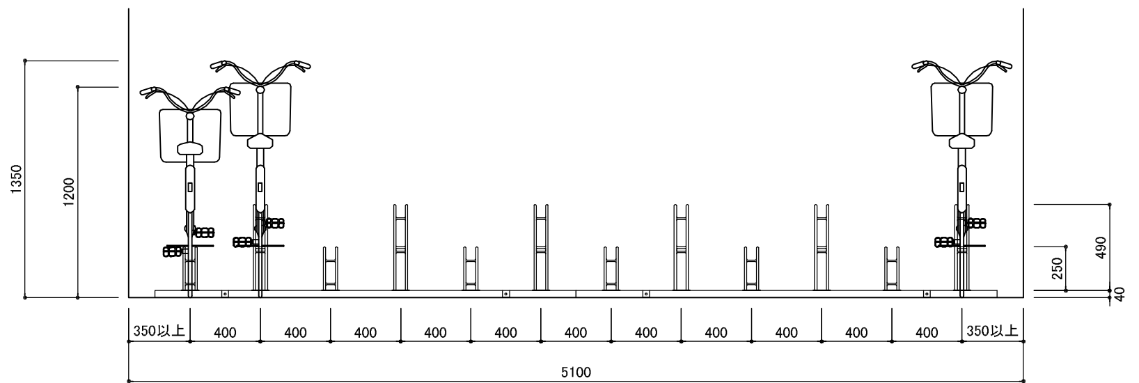
立面図 S=1/40
