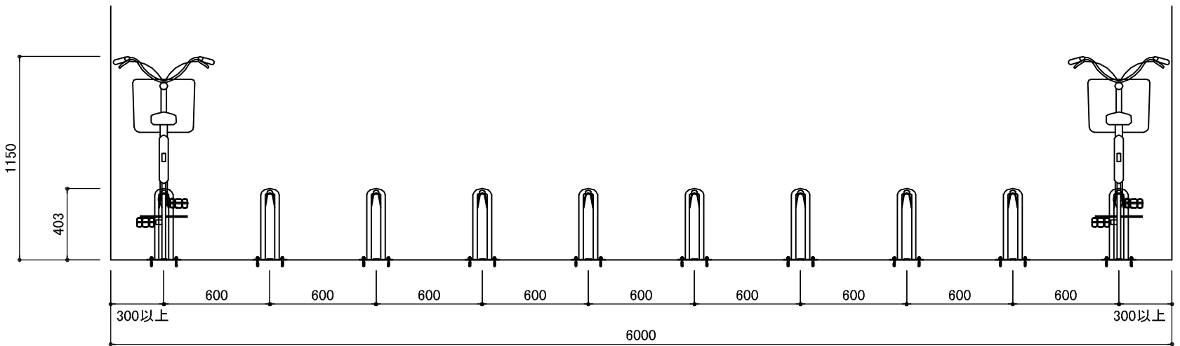
立面図 S=1/30
