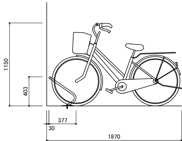
断面図 S=1/30
