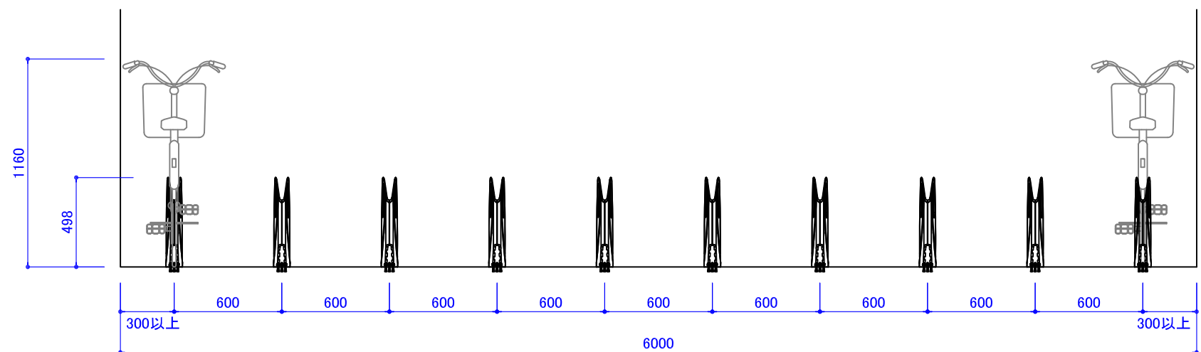
立面図
