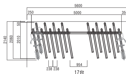
平面図 (10°)
