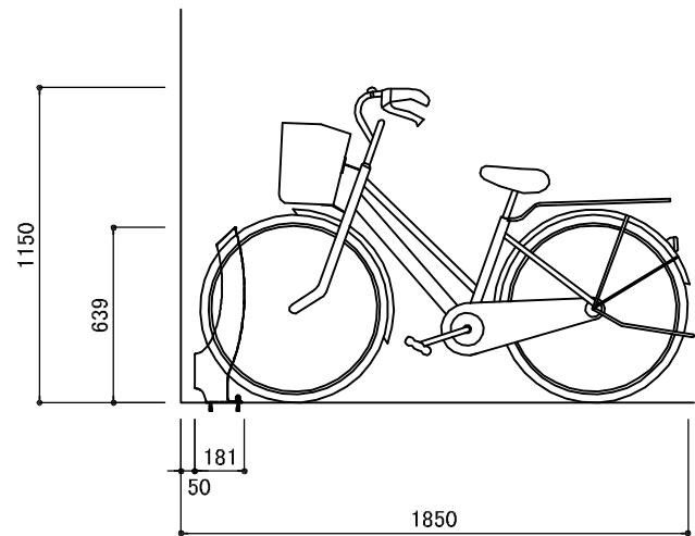
断面図 S=1/30
