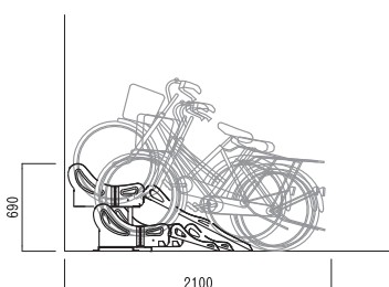
断面図
