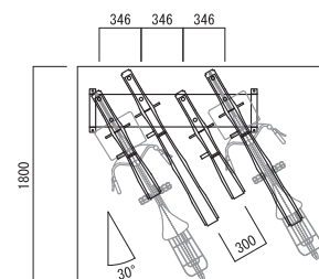
平面図 (30°)
