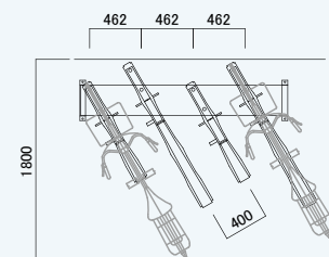
平面図 (30°)
