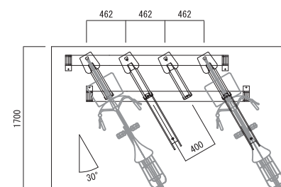
平面図 (30°)
