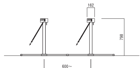
立面図
