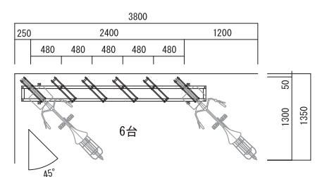
平面図 (45°)
