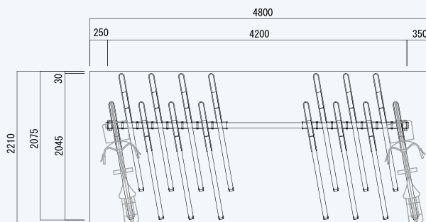
平面図 (10°)
