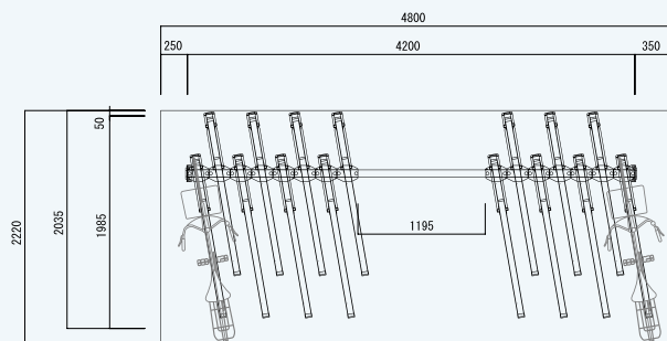
平面図 (10°)
