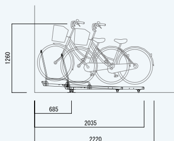
断面図
