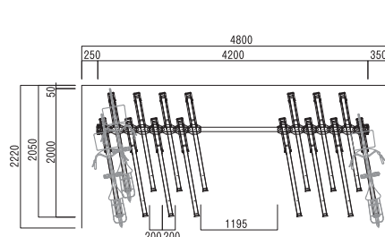
平面図 (10°)
