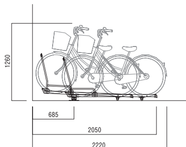
断面図
