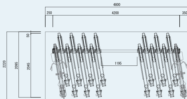
平面図 (10°)
