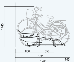
断面図
