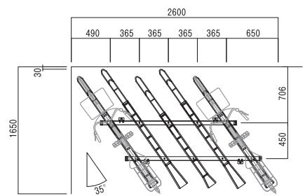
平面図 (35°)
