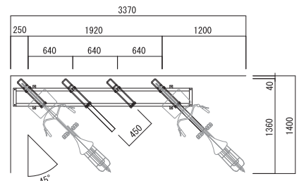
平面図 (45°)
