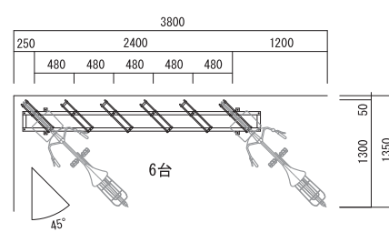
平面図 (45°)
