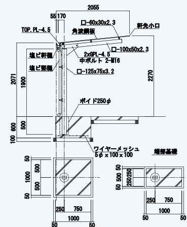
断面図
