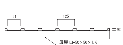
ガルバリウム角波鋼板詳細図
