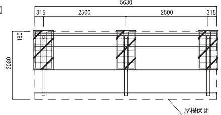
ガルバリウム角波鋼板詳細図
